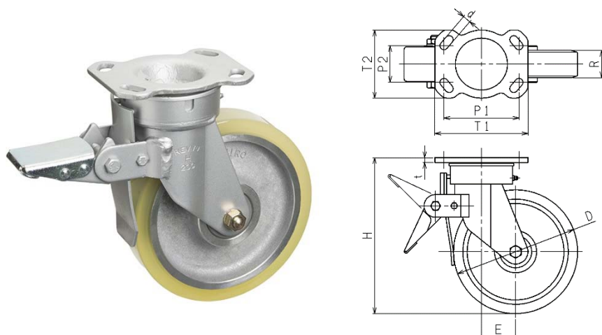
TSHB 型 (ストッパー付自由車)
