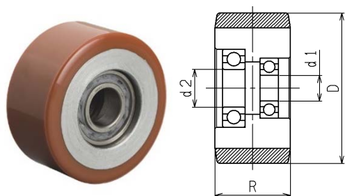
HPD 型（鉄製ホイールウレタン車輪）
