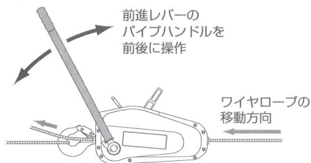
前進操作の場合
